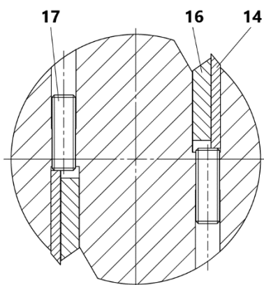
Рисунок 5. Схема регулировки строгальных ножей 14 – нож; 16 – прижимная планка; 17 – регулировочный винт
