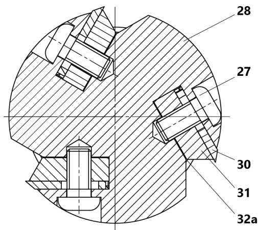
Рис. 10 Крепление ножей
