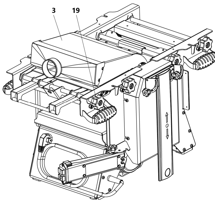
Рис. 7 Установка кожуха для удаления стружки при рейсмусовании 3 – кожух для удаления стружки; 19 – гайка-барашек
