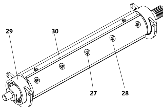
Рис. 9 Конструкция ножевого вала 27 – зажимной винт; 28 – вал ножевой; 29 – подшипниковый узел; 30 – нож
