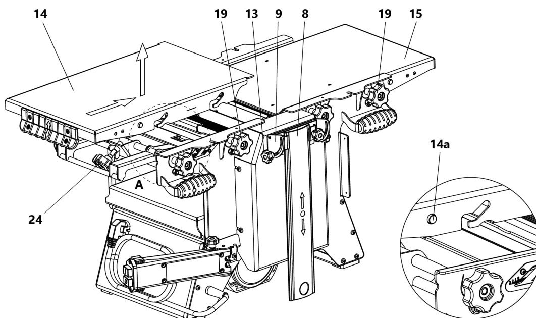
Рис. 6 Снятие приемного и загрузочного строгальных столов со станка
