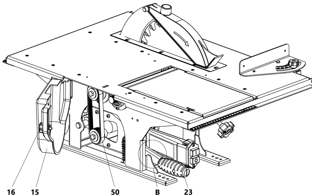
Рисунок 12. Установка приводного ремня 15 – кожух защиты ремня, 16 – винт-барашек, 23 – ручка, 50 – ремень
