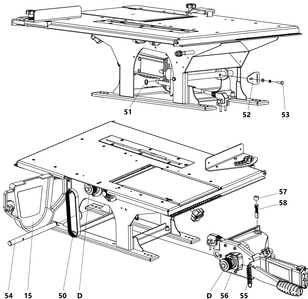
Рисунок 13. Схема разборки станка при замене щеток
